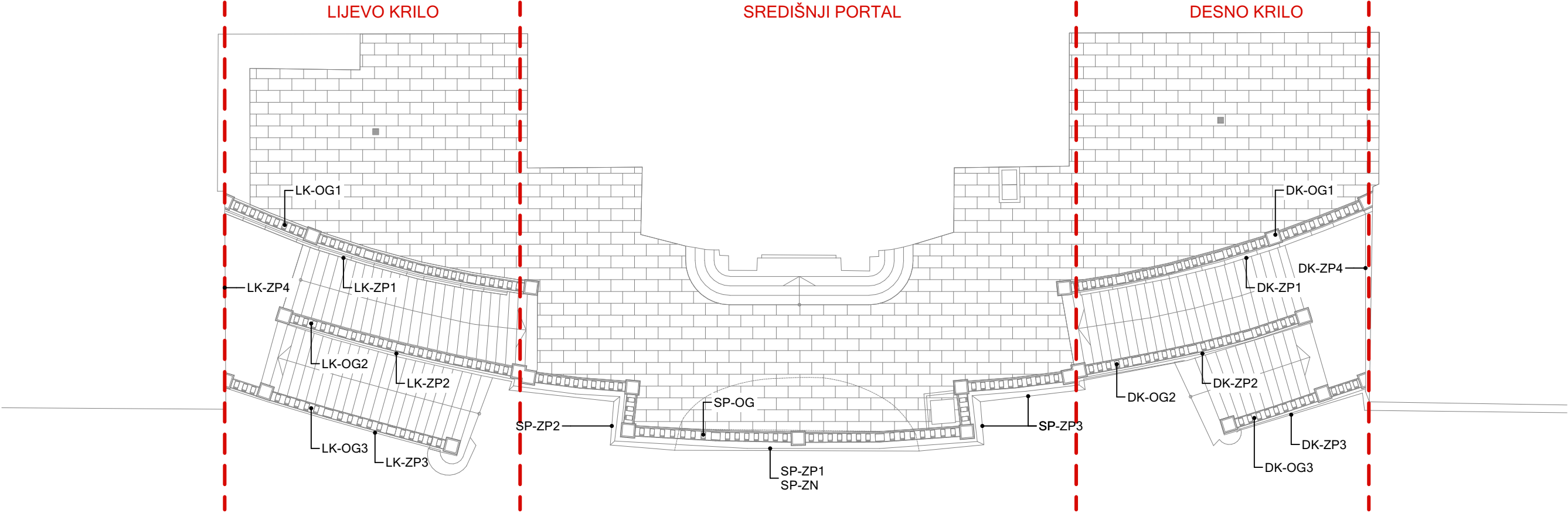
TLOCRT ULAZNOG PLATOA M 1:150
