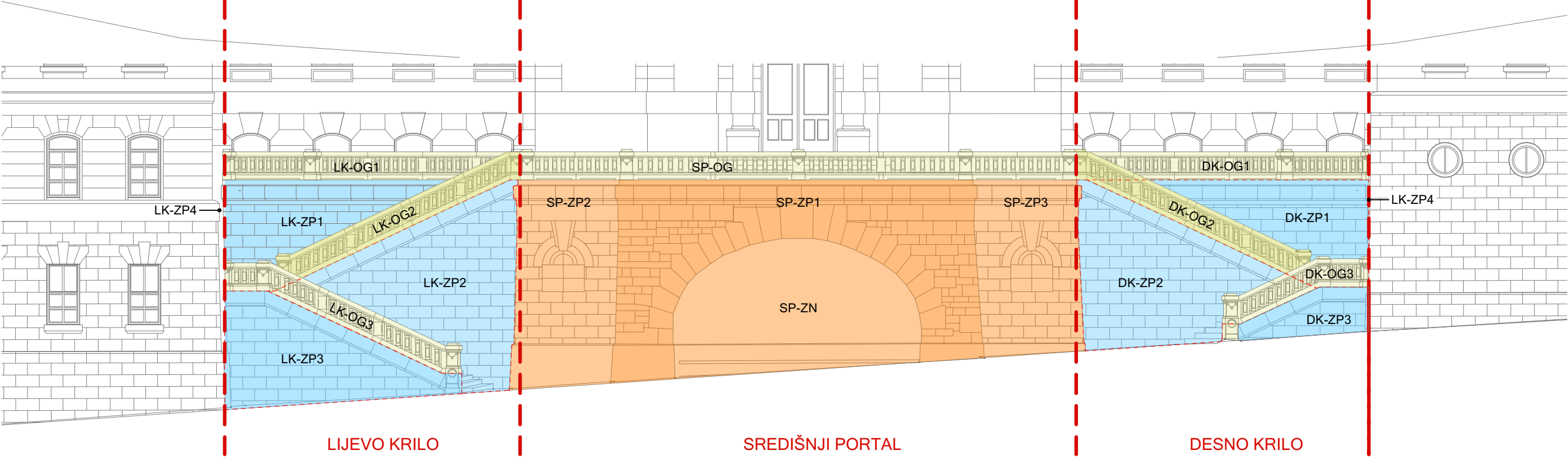
PROČELJE ULAZNOG PLATOA M 1:150
